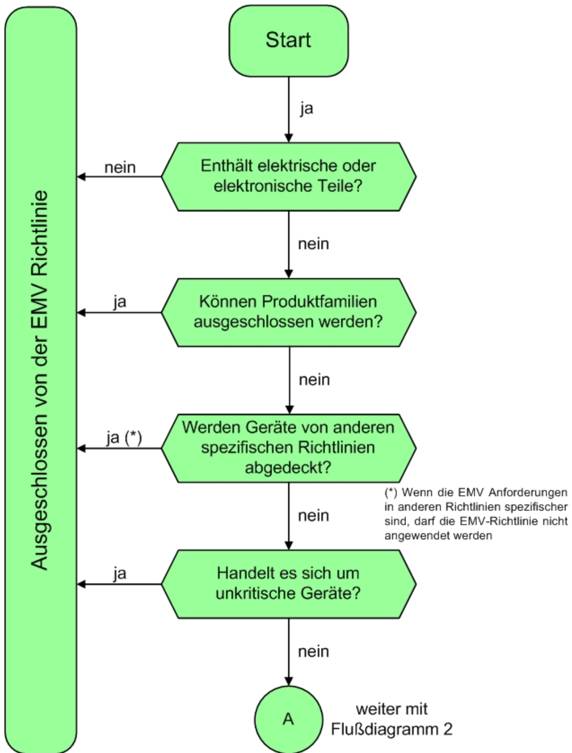
Ablaufdiagramm 1 – Anwendungsbereich
